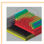
Disipador incorporado
