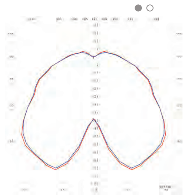
Curva fotométrica LED 60w
