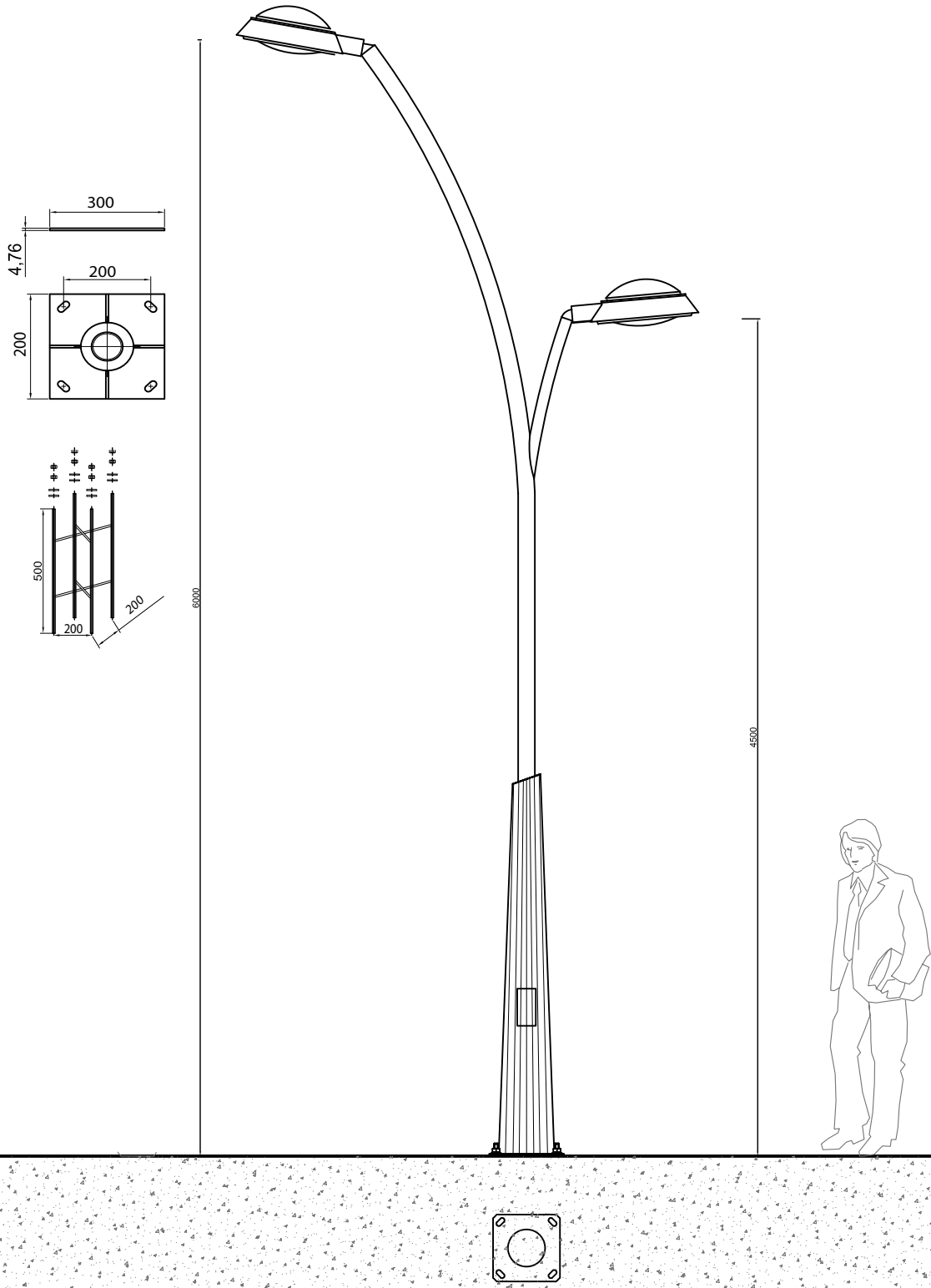
PERNOS DE ANCLAJE CRUCETA M18X500
